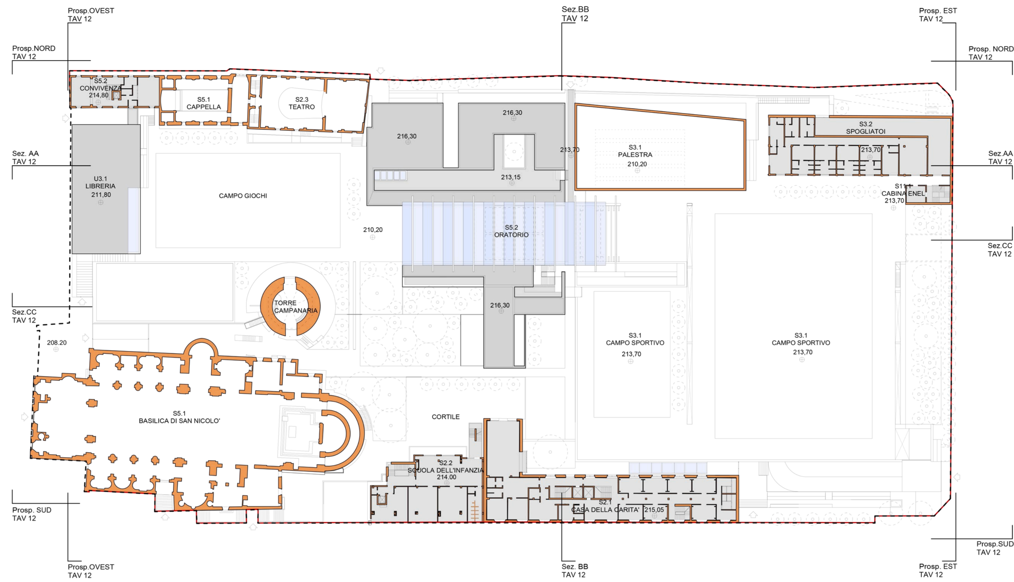
LIVELLO +1 (quota +216,00)
