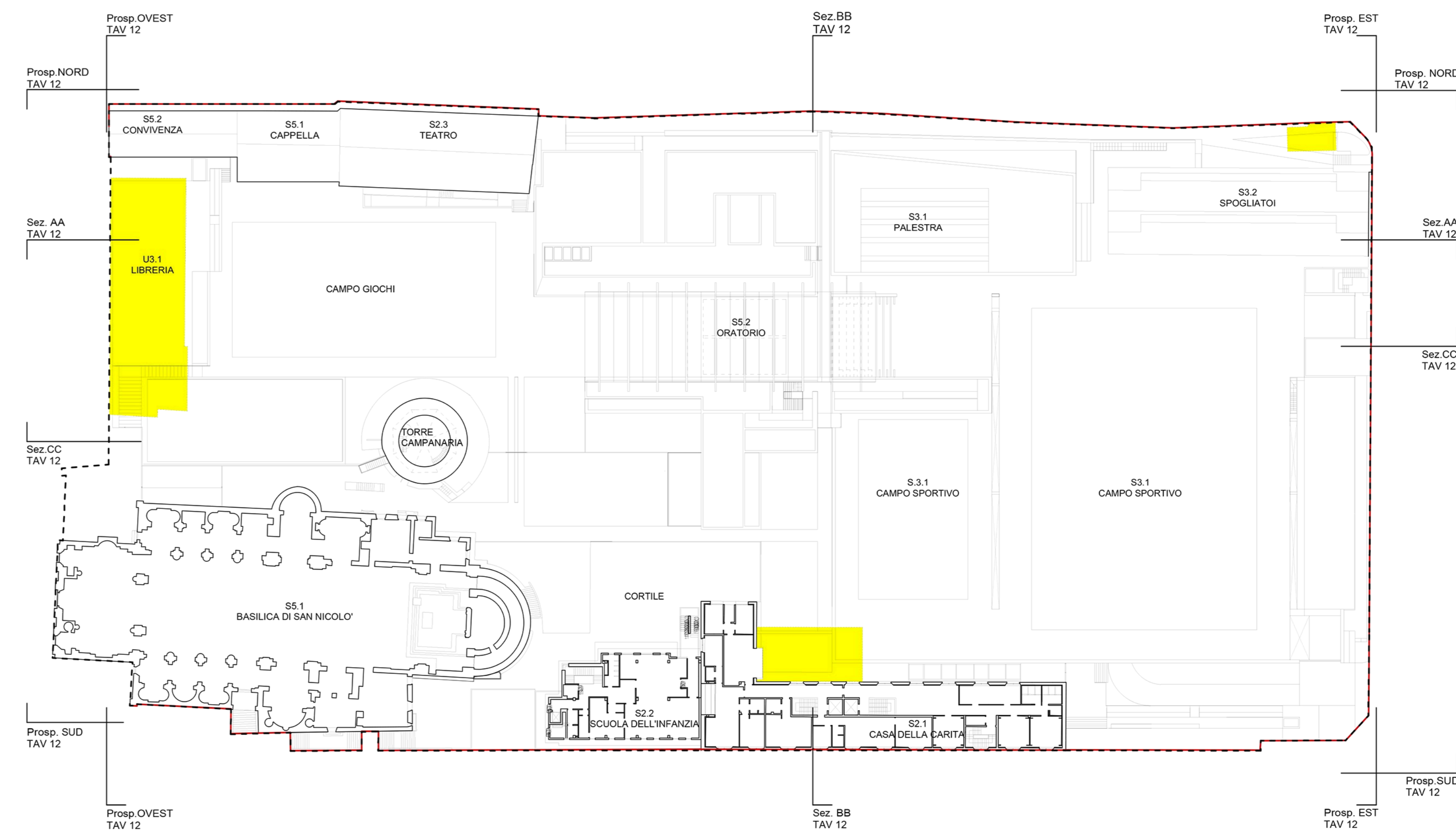
LIVELLO +2 (quota +220,00)
