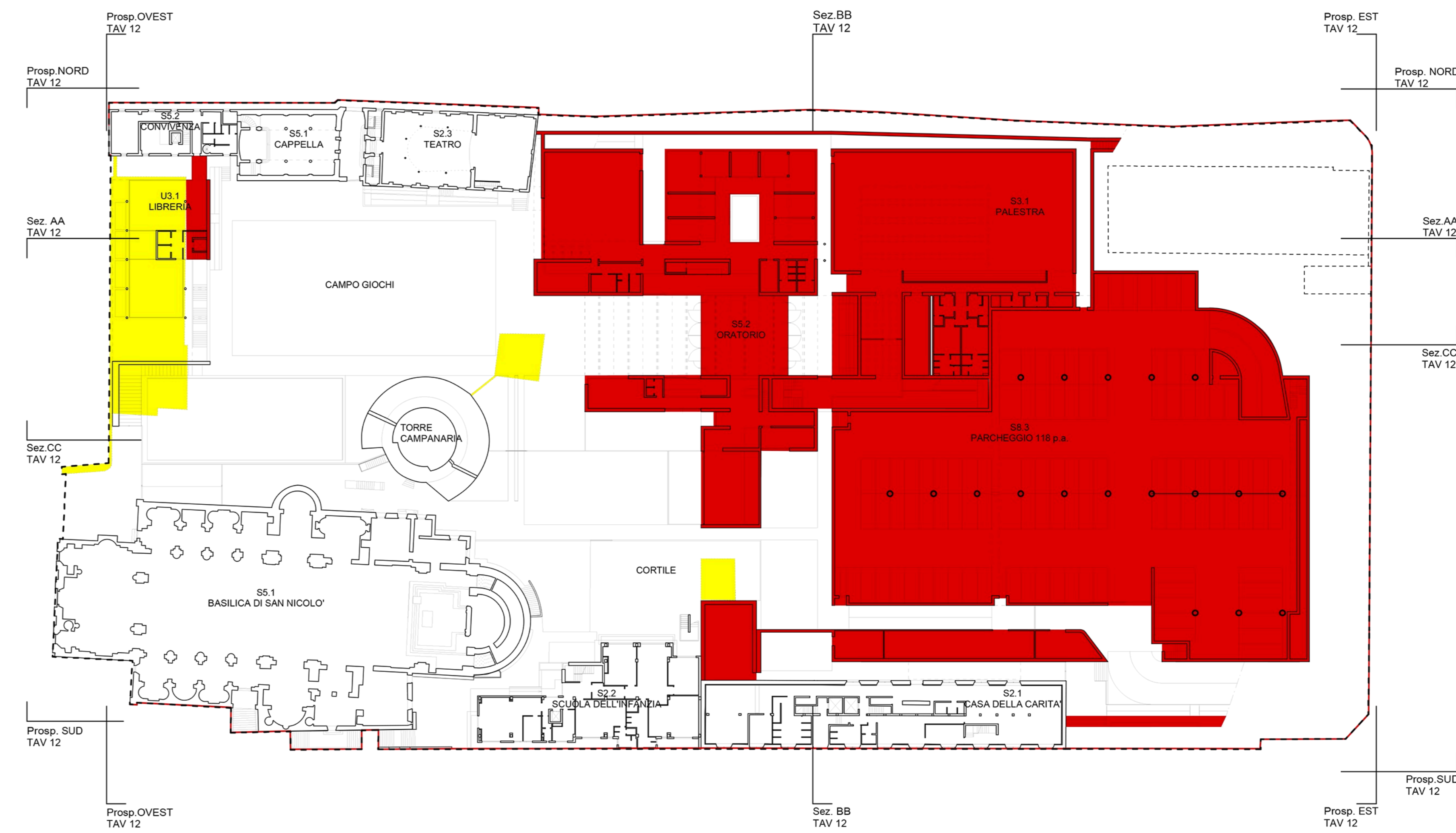
LIVELLO 0 (quota +211,00)
