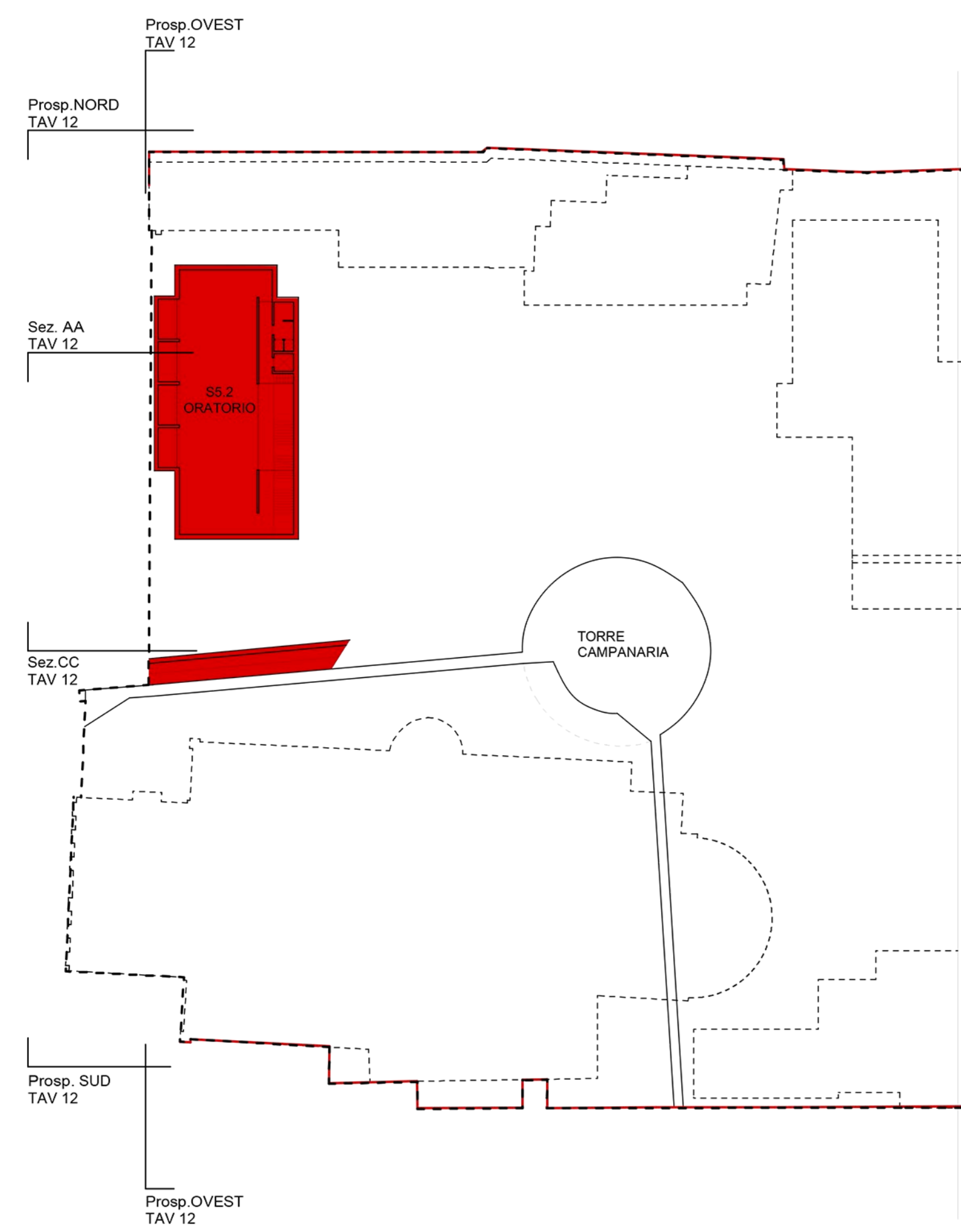
LIVELLO -2 (quota +203,00)
